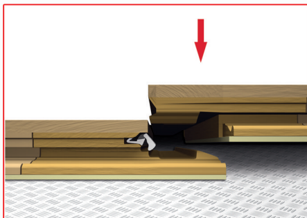
Metoda 1: Spouštění Method 1: Drop down
