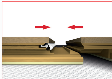
Metoda 3: Horizontální zasunutí Method 3: Horizontal insertion
