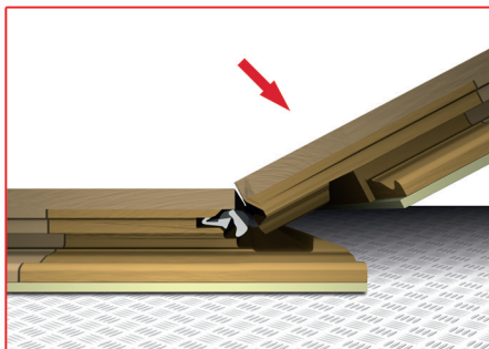
Metoda 2: Pokládání pod úhlem Method 2: Angling
